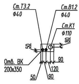
Типовое расположение стоек в отверстиях 200x350
