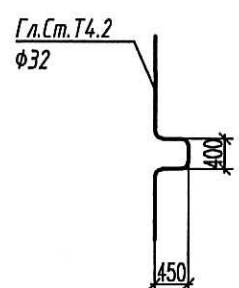
При расположении 1 стойки
