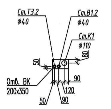
Типовое расположение стояков в отверстиях 200x350
