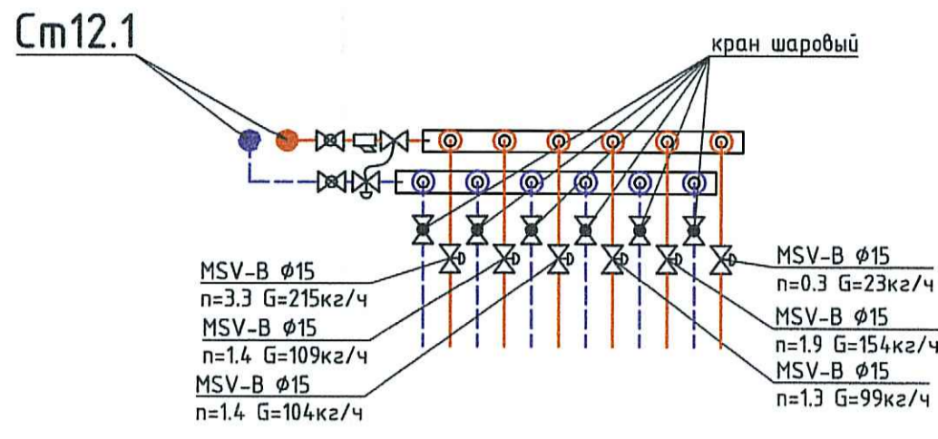
Коллектор 12.1.3-12.1.9
