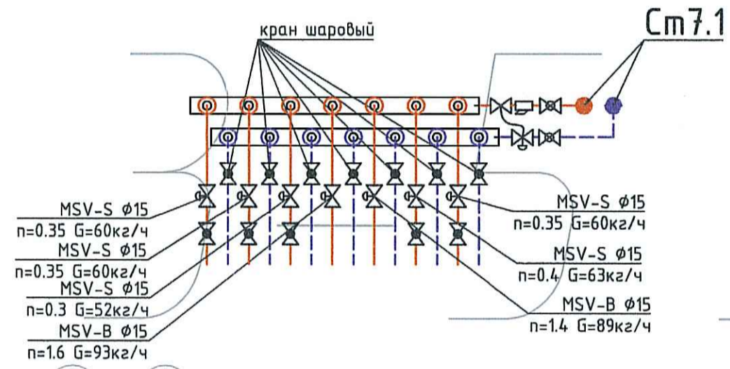
Коллектор 7.1.3-7.1.9
