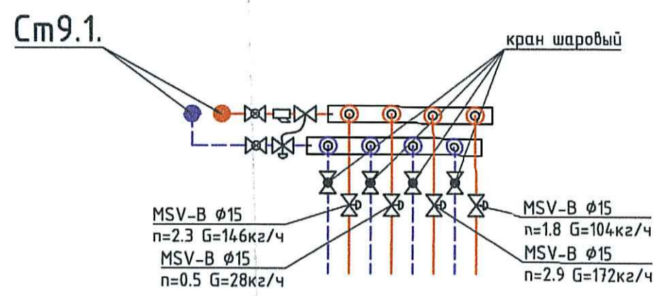
Коллектор 9.1.3-9.1.9
