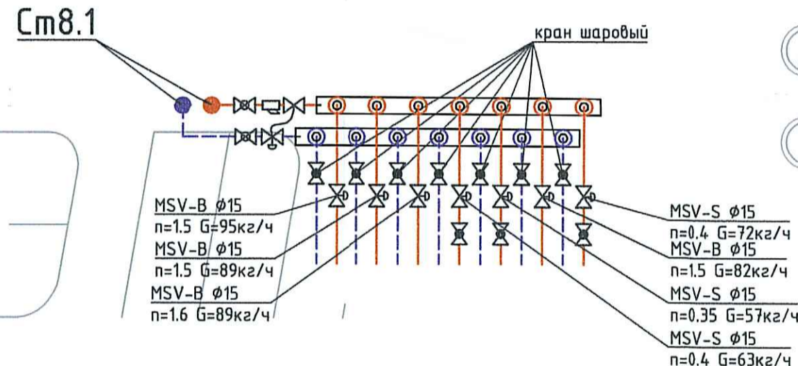
Коллектор 8.1.3-8.1.9
