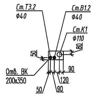
Типовое расположение стояков в отверстии 200x350
