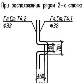
П-образные компенсаторы для главных стояков систем Т4.1 и Т4.2 предусматриваются на 3, 6, 9, 12 и 15 этажах
