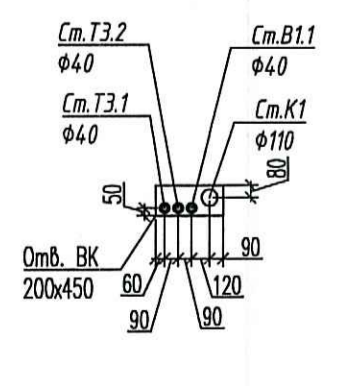
Типовое расположение стояков в отверстиях 200x450
