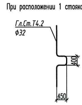
П-образные компенсаторы для главных стояков систем Т4.1 и Т4.2 предусматриваются на 3, 6, 9, 12 и 15 этажах
