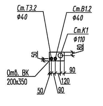
Типовое расположение стояков в отверстии 200х350
